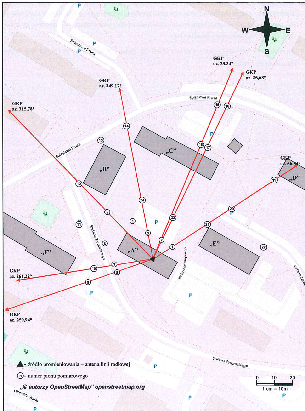
Rys. 1. Usytuowanie punktów i pionów pomiarowych w otoczeniu instalacji radiokomunikacyjnej Stacja Netia LOMZB006-LOMZM00052 Łomża, ul. Stefana Żeromskiego 1
